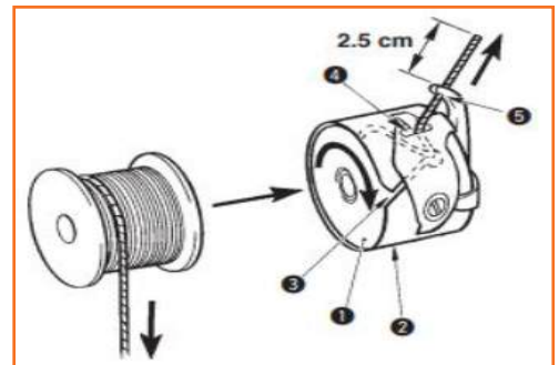
Fig.2.4.19: Installing bobbin
